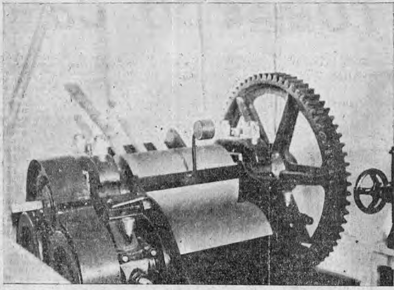
TRAPICHE para moler dos y media toneladas de azúcar por hora, fabricado por PINTO & CARAZO. Mas de cien trapiches de diversos tamaños y potencialidad, fabricados en esa gran fábrica de implementos agrícolas se encuentran en servicio en casi todas las regiones del país, siendo la mejor recomendación de la alta calidad y perfeccionamiento de esas maquinarias de fabricación Nacl.
