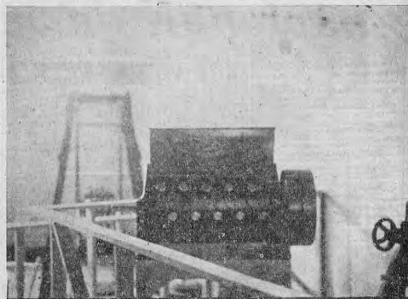
MAGNIFICA CHANCRADORA de café construí en los talleres de PINTO & CARAZO, considerada como una de las maquinarias más perfectas y que en nada tiene que envidiar a las mejores fabricadas en el extranjero
