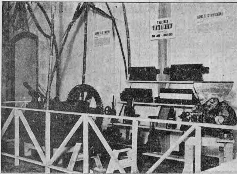
STAND de los grandes talleres de fundición y mecánica de PINTO & CARAZO mostrando parte de la maquinaria para beneficiar café y otros productos
